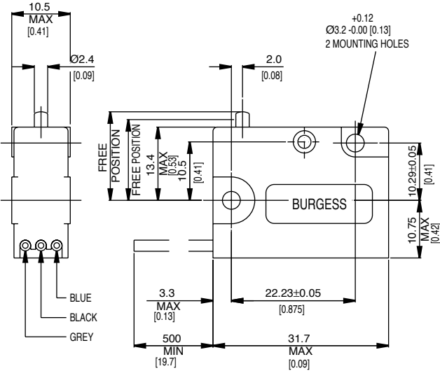
Dimensions
