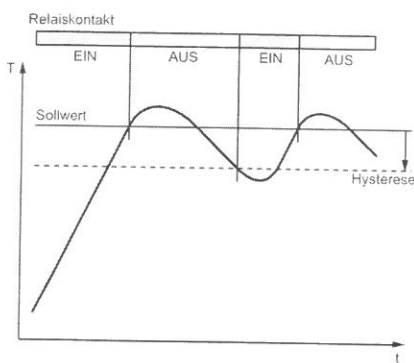
Heizregler, einseitige Hysterese
