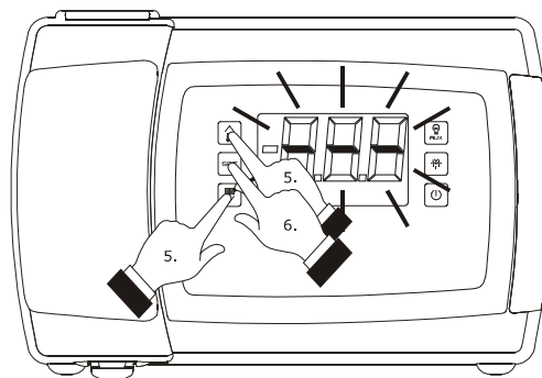
Cancellazione delle ore di funzionamento del compressore
