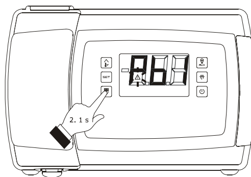
Accesso alla procedura per la cancellazione delle ore di funzionamento del compressore
