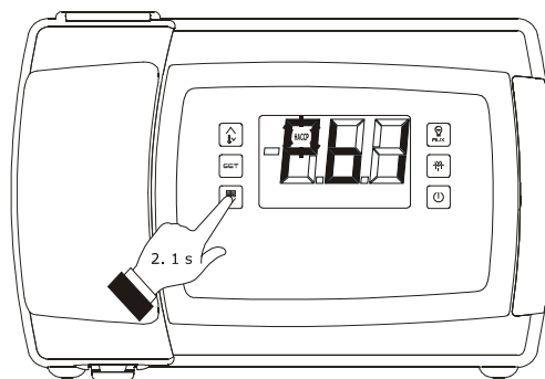
Accesso alla procedura per la cancellazione delle informazioni riguardanti gli allarmi HACCP
