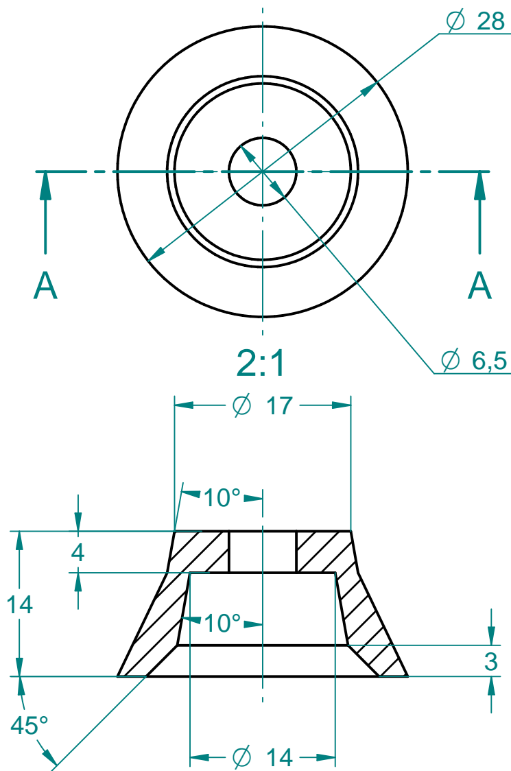
CORTE A-A
