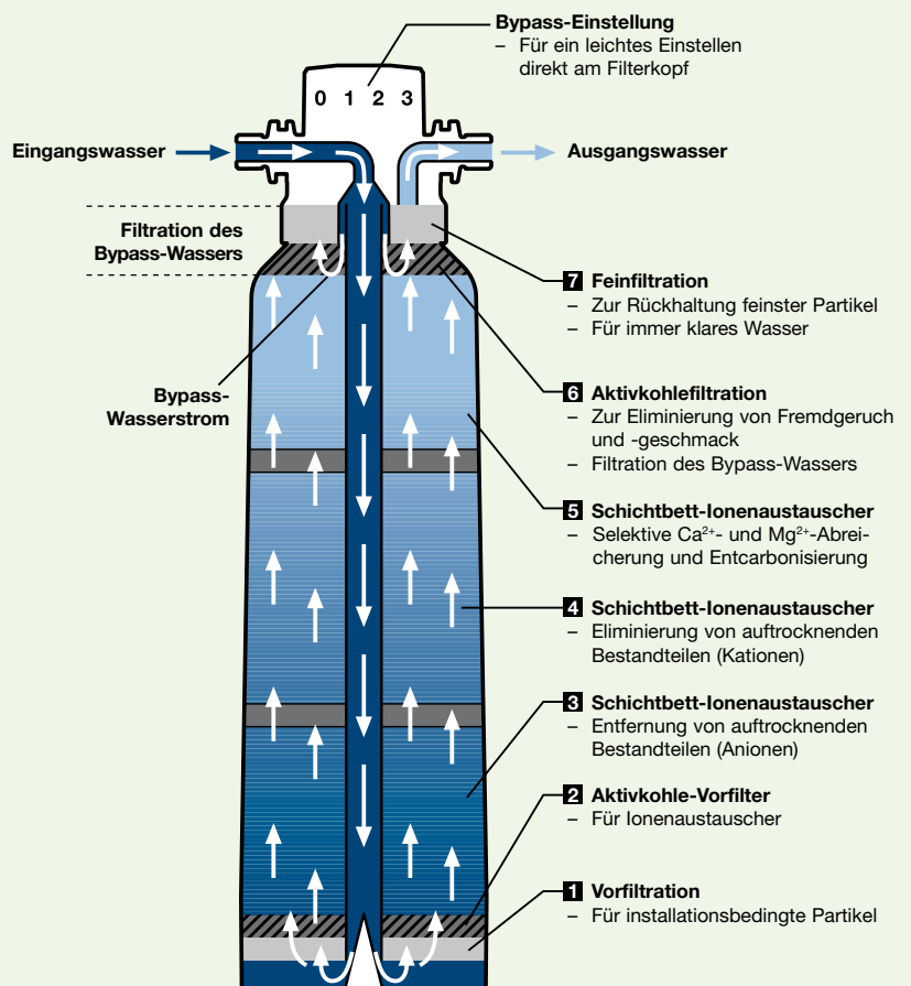
Aufbau einer BWT bestclear EXTRA Filterkerze mit 7-fach-Filtration
