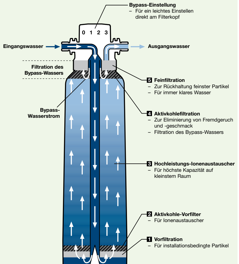
Aufbau einer BWT bestclear Filterkerze mit 5-fach-Filtration
