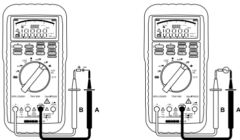
Bild 4: Gleichstrommessung Fig. 4: DC current measurement Fig. 4: Mesure de courant continu Fig. 4: Medición de corriente continua obr. 4: Měření stejnosměrného proudu σχήμα 4: DC- μέτρηση ill. 4: Misura corrente continua Fig. 4: Meten van gelijkstroom Rys. 4: Pomiar prądu stałego рис. 4: Измерение постоянного тока Fig. 4: Likströmsmätning Resim 4: Doğru Akım Ölçümü Bild 5: Wechselstrommessung Fig. 5: AC current measurement Fig. 5: Mesure de courant alternatif Fig. 5: Medición de corriente alterna obr. 5: Měření střídavého proudu σχήμα 5: AC- μέτρηση ill. 5: Misura corrente alternata Fig. 5: Meten van wisselstroom Rys. 5: Pomiar prądu przemiennego рис. 5: Измерение переменного тока Fig. 5: Växelsrömsmätning Resim 5: Alternatif Akım Ölçümü
