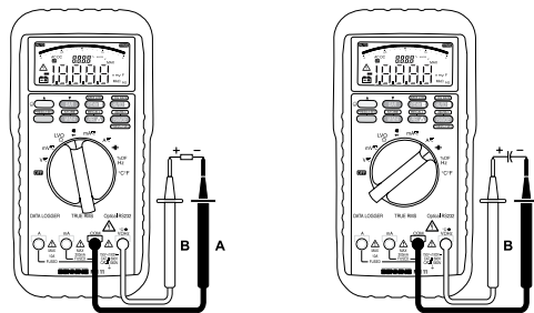
Bild 8: Durchgangsprüfung mit Summer Fig. 8: Continuity Testing with buzzer Fig. 8: Contrôle de continuité avec ronfleur Fig. 8: Control de continuidad con vibrador obr. 8: Zkouška obvodu σχήμα 8: Έλεγχος συνέχειας με βομβητή ill. 8: Prova di continuità con cicalino Fig. 8: Doorgangstest met akoestisch signaal Rys. 8: Sprawdzanie ciągłości obwodu рис. 8: Проверка прохождения тока с зуммером Fig. 8: Genomgångstest med summer Resim 8: Sesli Uyarıcı ile Süreklilik Kontrolü Bild 9: Kapazitätsmessung Fig. 9: Capacity Testing Fig. 9: Mesure de capacité Fig. 9: Medición de capacidad obr. 9: Měření kapacity σχήμα 9: Μέτρηση χωρητικότητας ill. 9: Misura di capacità Fig. 9: Capaciteitsmeting Rys. 9: Pomiar pojemności рис. 9: Измерение емкости Fig. 9: Kapacitansmätning Resim 9: Kapasite Ölçümü
