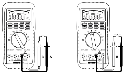
Bild 6: Widerstandsmessung Fig. 6: Resistance measurement Fig. 6: Mesure de résistance Fig. 6: Medición de resistencia obr. 6: Měření odporu σχήμα 6: Μέτρηση αντίστασης ill. 6: Misura di resistenza Fig. 6: Weerstandsmeting Rys. 6: Pomiar rezystancji рис. 6: Измерение сопротивления Fig. 6: Resistansmätning Resim 6: Direnç Ölçümü Bild 7: Diodenprüfung Fig. 7: Diode Testing Fig. 7: Contrôle de diodes Fig. 7: Verificación de diodos test diod σχήμα 7: Έλεγχος διόδου. ill. 7: Prova diodi Fig. 7: Diodecontrole Rys. 7: Pomiar diody рис. 7: Проверка диодов Fig. 7: Diod-test Resim 7: Diyot Ölçümü
