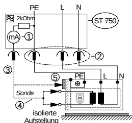
Berührungsstrommessung: DIN VDE 0701-0702 (Sk I) mit Stromausg.
