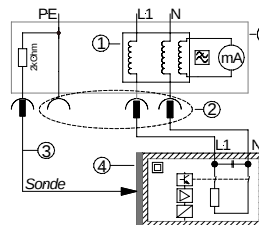
Berührungsstrommessung: DIN VDE 0701-702 (Sk I-II)
