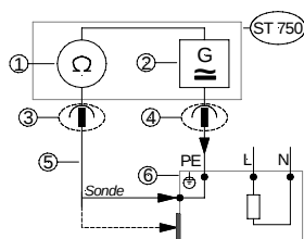
Schutzleiterprüfung R_{PE} : DIN VDE 0701-0702 (SK I)
