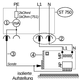
Geräteableitstrommessung / Direktmessung: DIN VDE 0751-1 (Sk II)
