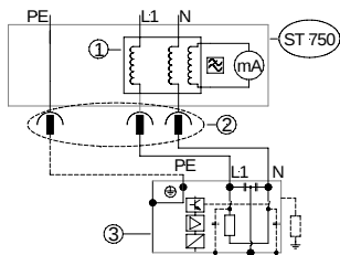
Schutzleiterstrommessung / Differenzstromverfahren: DIN VDE 0701-702 (Sk I-II)
