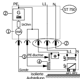
Ableitstrom vom Anwendungsteil, Netzspg. am AP, Typ F – direkte Messung: DIN VDE 0751-1 (Sk I)
