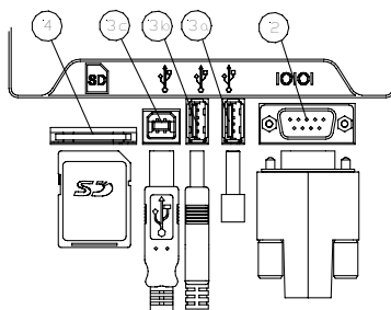
Ansicht Anschlussseite:
