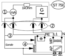
Ableitstrom vom Anwendungsteil des Typs F – Ersatzableitstrommessung: DIN VDE 0751-1 (SK I)
