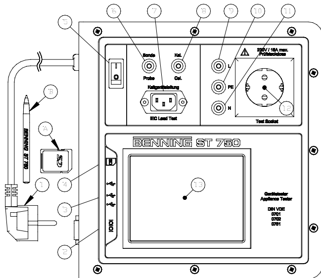
Ansicht Anschlussseite:
