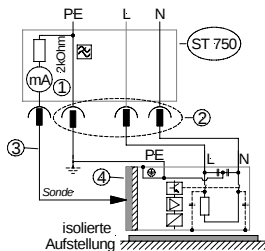
Berührungsstrommessung: DIN VDE 0701-0702 (Sk I)
