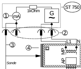
Geräteableitstrom / Ersatzableitstrommessung: DIN VDE 0751-1 (SK II)
