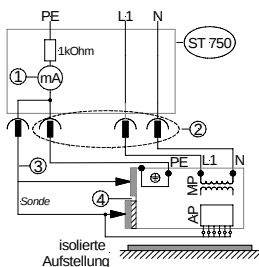
Geräteableitstrommessung / Direktmessung: DIN VDE 0751-1 (Sk I)
