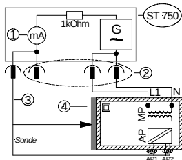
Ableitstrom vom Anwendungsteil des Typs F – Ersatzableitstrommessung: DIN VDE 0751-1 (SK II)
