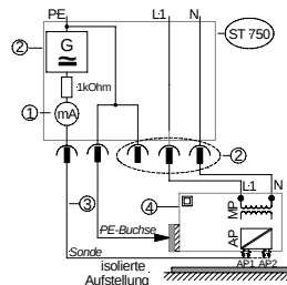
Ableitstrom vom Anwendungsteil, Netzspg. am AP, Typ F – direkte Messung: DIN VDE 0751-1 (Sk II)
