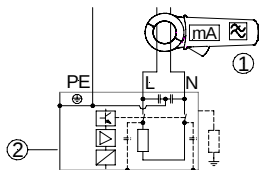
Schutzleiterstrommessung / Differenzstromverfahren: DIN VDE 0701-702 (Sk I-II)
